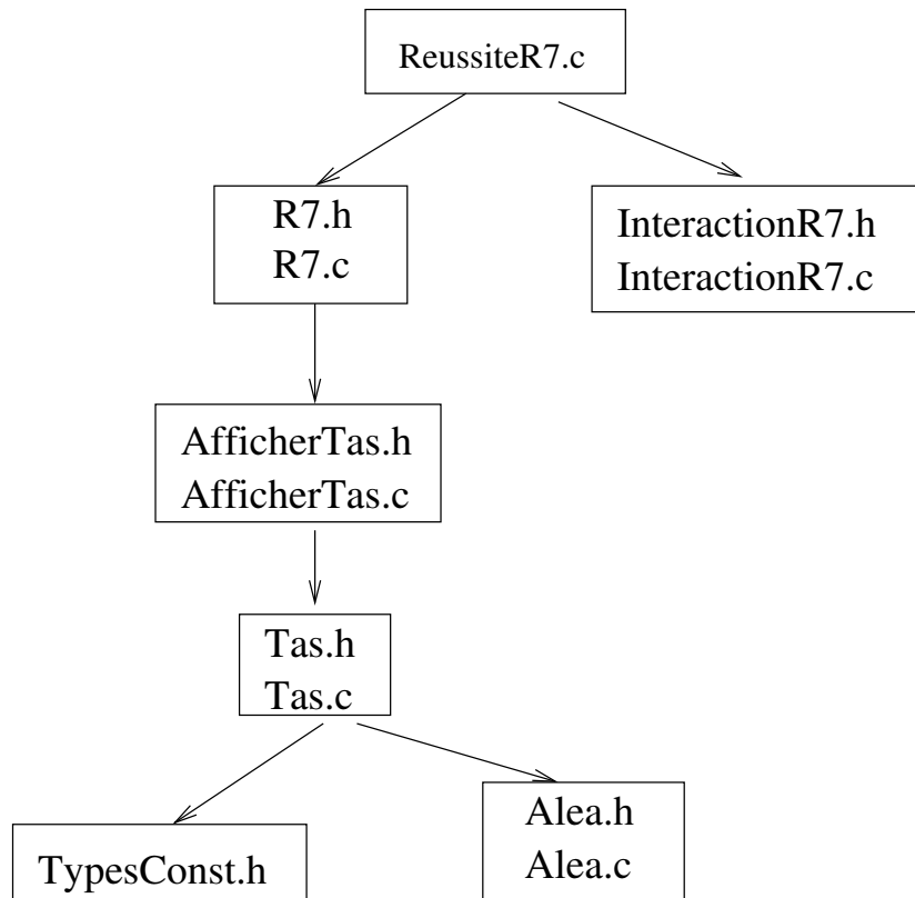
FIGURE 1 – Dépendance entre les fichiers C fournis
